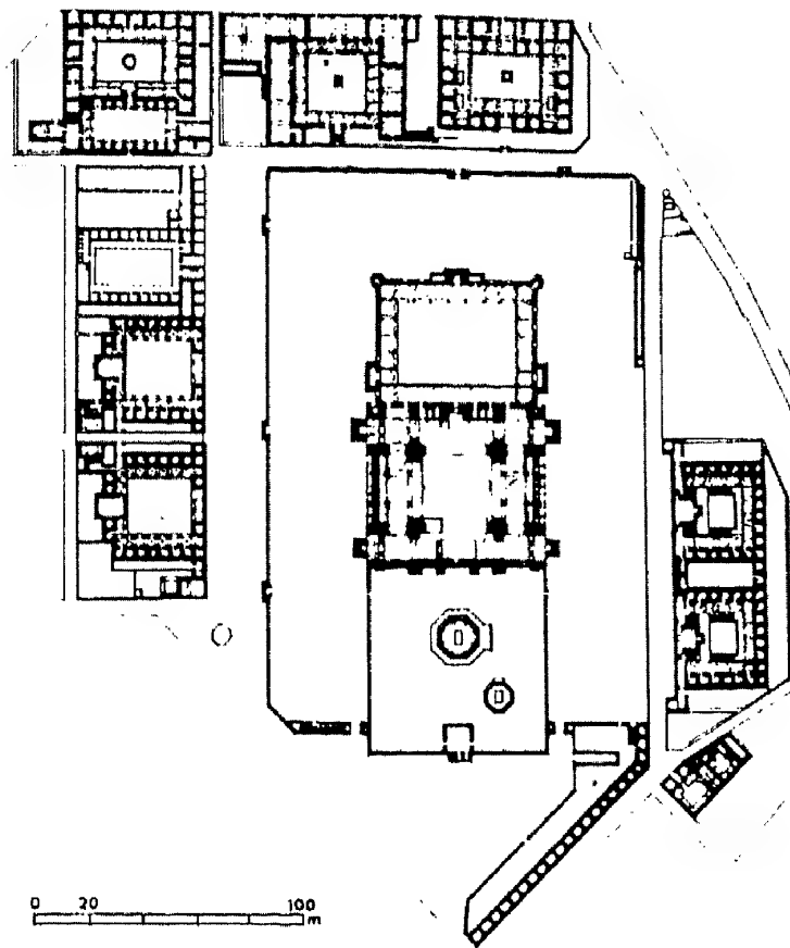
الشكل ٢٢ - ١٠ مجمّع السليمانية، اسطيول (١٥٥٠ - ١٥٥٧م)
